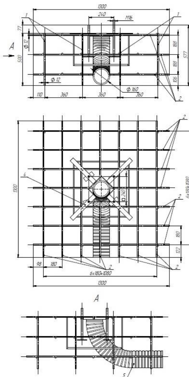
Рисунок 5.3 Схема з розмірами армування та складових бетонної основи
