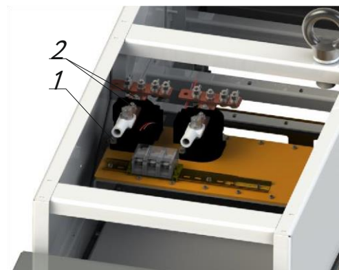
Рисунок 7.8. Реле постійного струму
