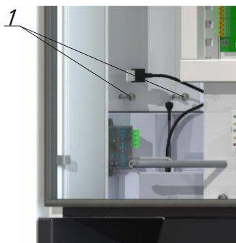
Рисунок 7.10 Кріплення екрану
