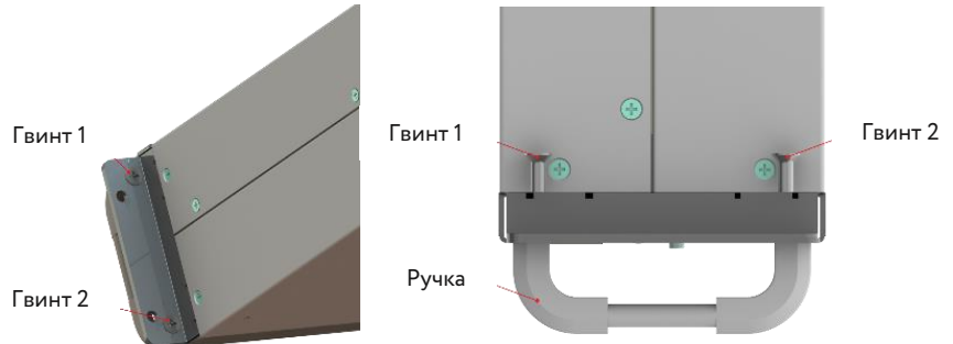
Рисунок 5.11. Розташування кріплень
