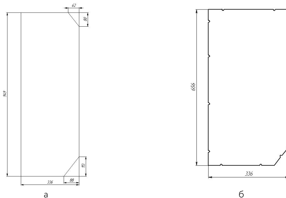
Рисунок 7.2 Розміри фільтруючих елементів
