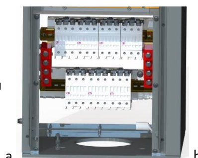
Рисунок 7.5 Відсік реле та шин
