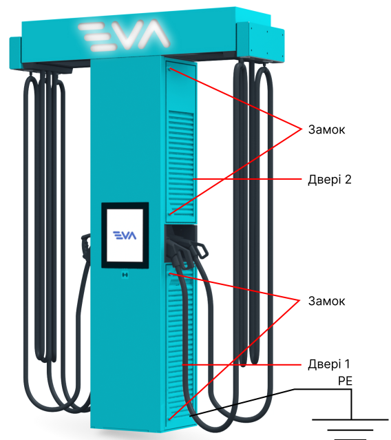
Рисунок 5.12. Розташування дверей та замків
